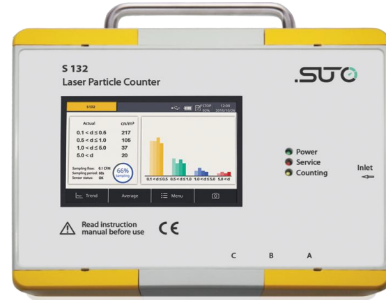
Partikül Sayacı
